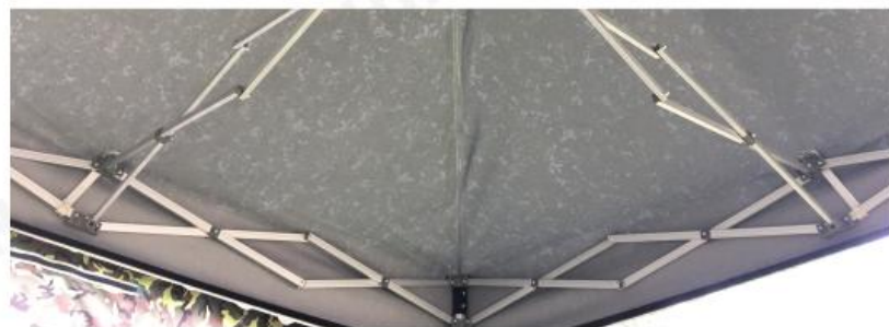
A 上角柱 B 交叉管 C 頂柱 D 固定勾
